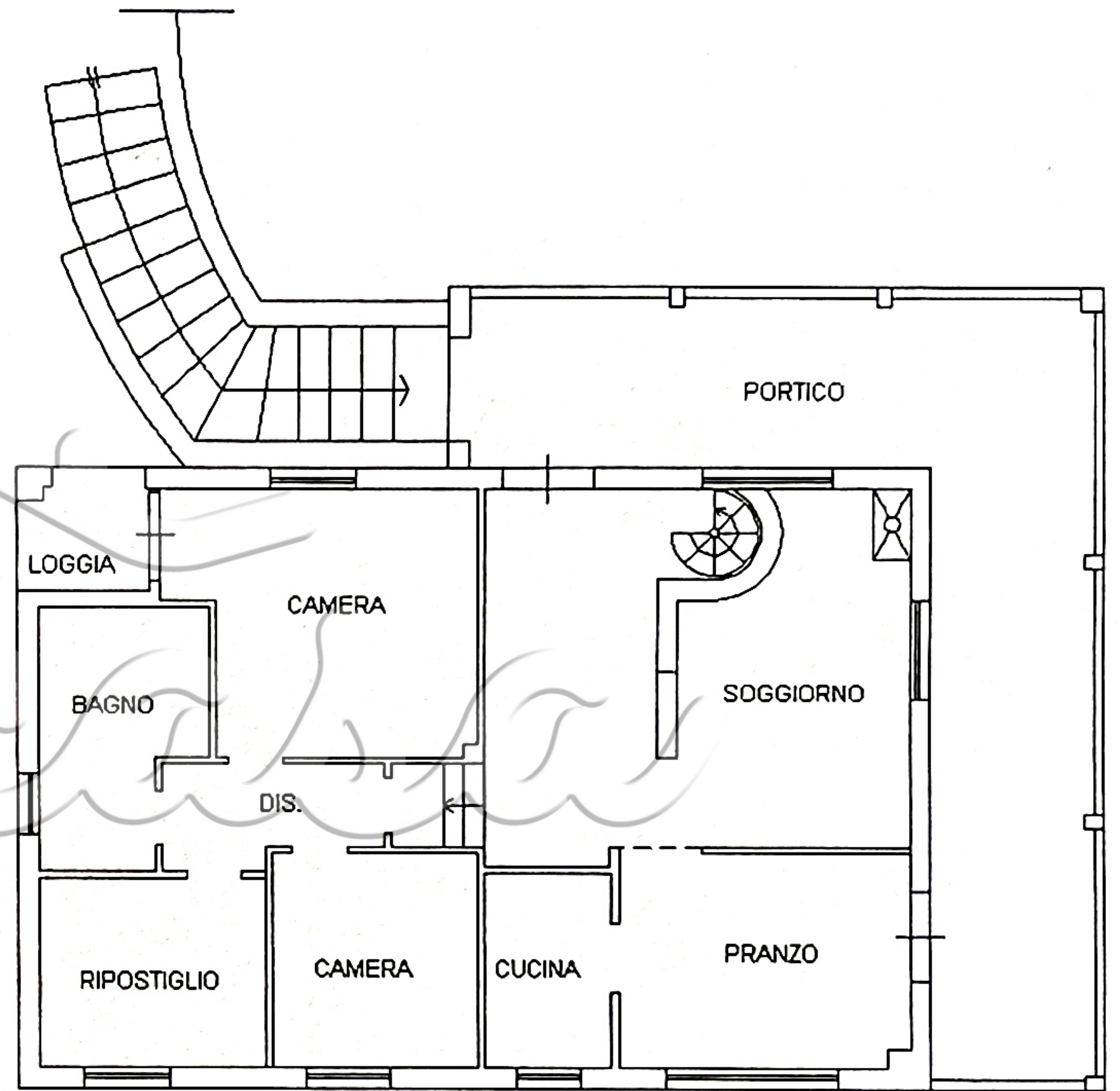
PIANO PRIMO H. 3,00
