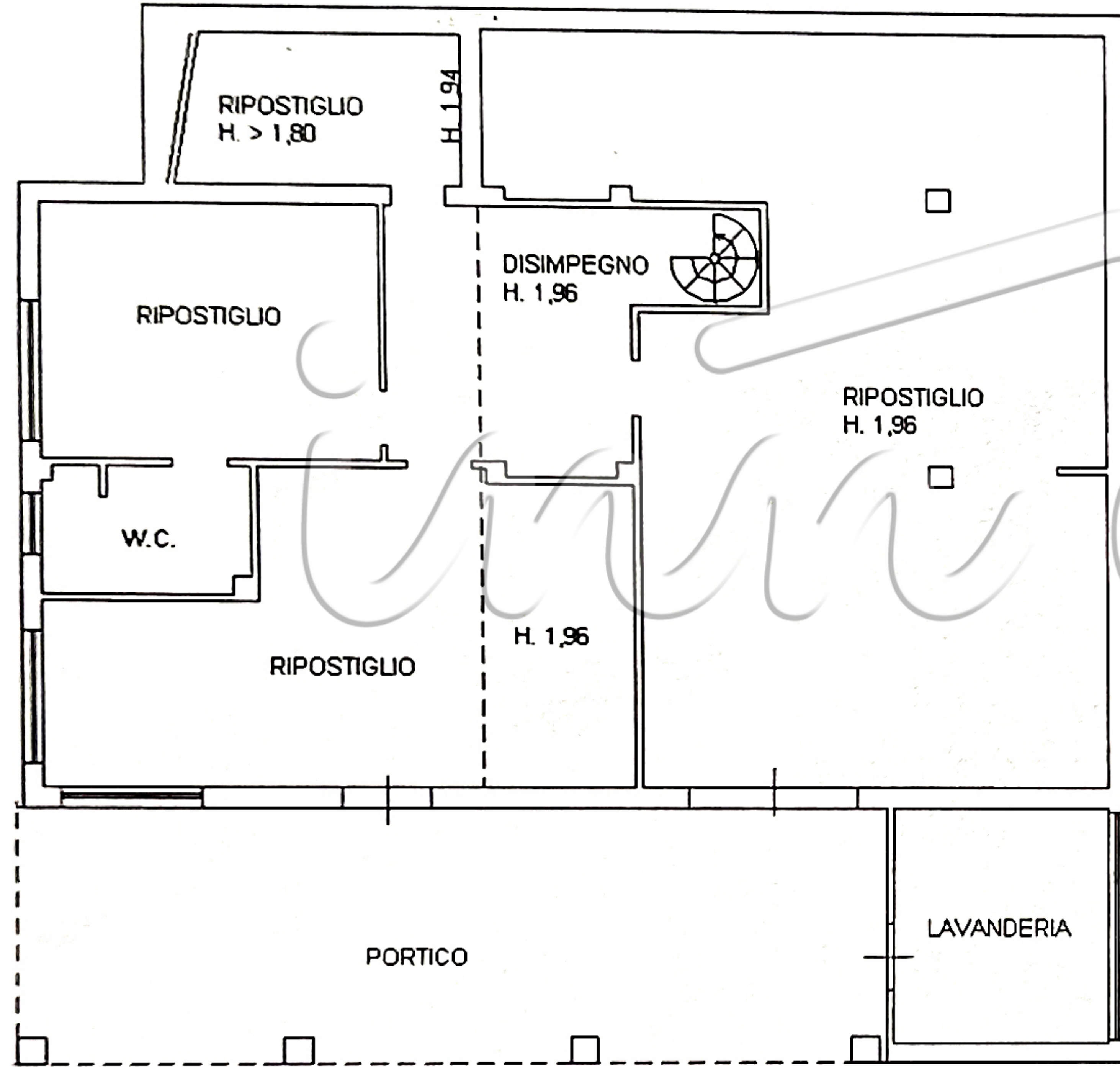
PIANO TERRA H. 2,50
